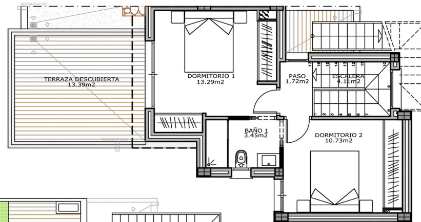
PLANTA PRIMERA
