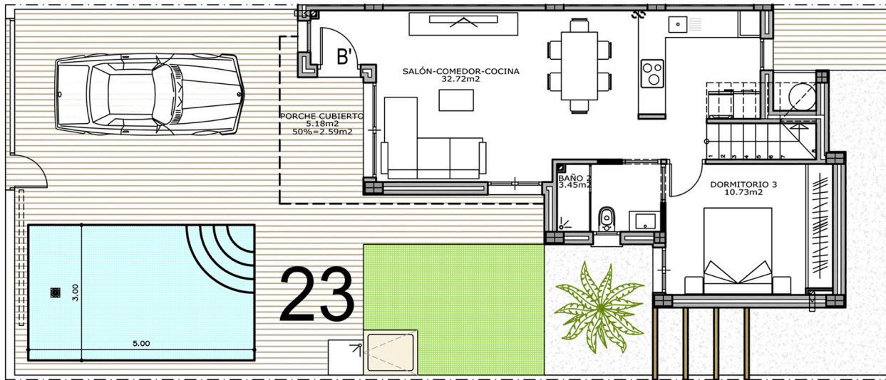
PLANTA BAJA
